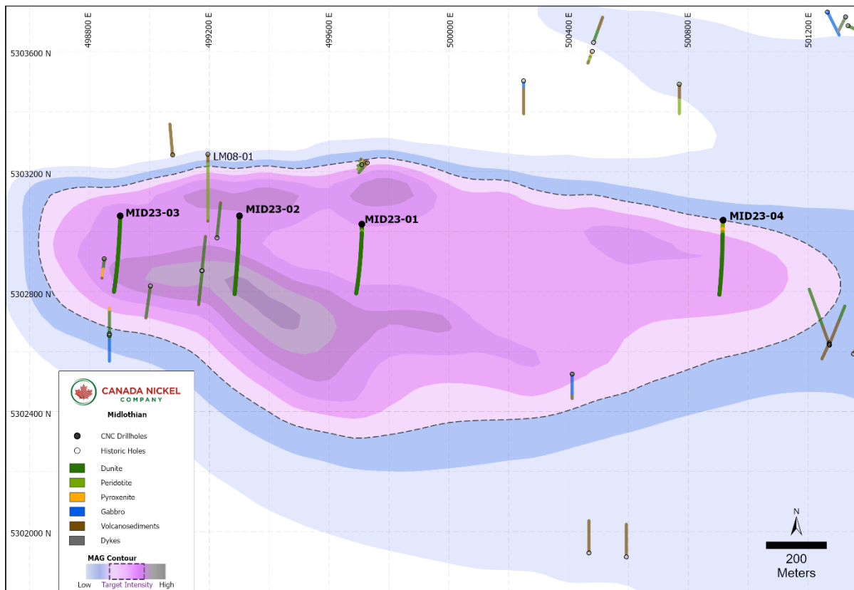
Abbildung 1 - Planansicht von Midlothian - aktuelle und historische Bohrungen überlagert mit der magnetischen Gesamtintensität
