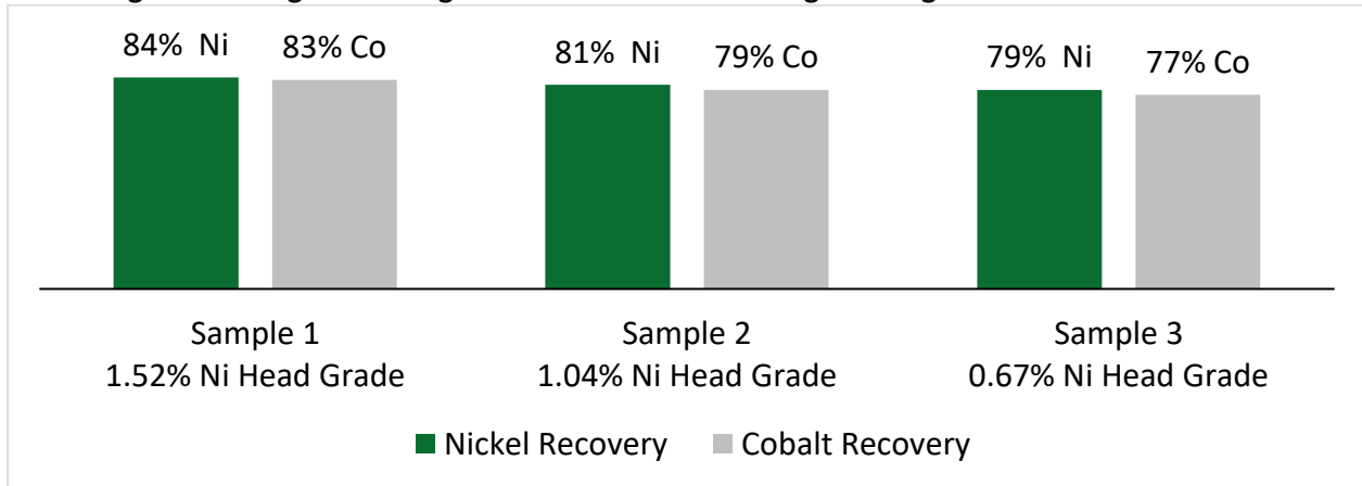
Abbildung 1. Vorläufige metallurgische Arbeiten - Gewinnungsleistung von Texmont
