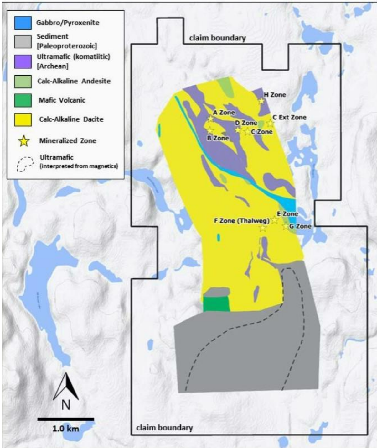
Abbildung 2 - Grundstück Bannockburn mit Nickel-Sulfid-Zonen (modifiziert nach Outokumpu, 1999).
