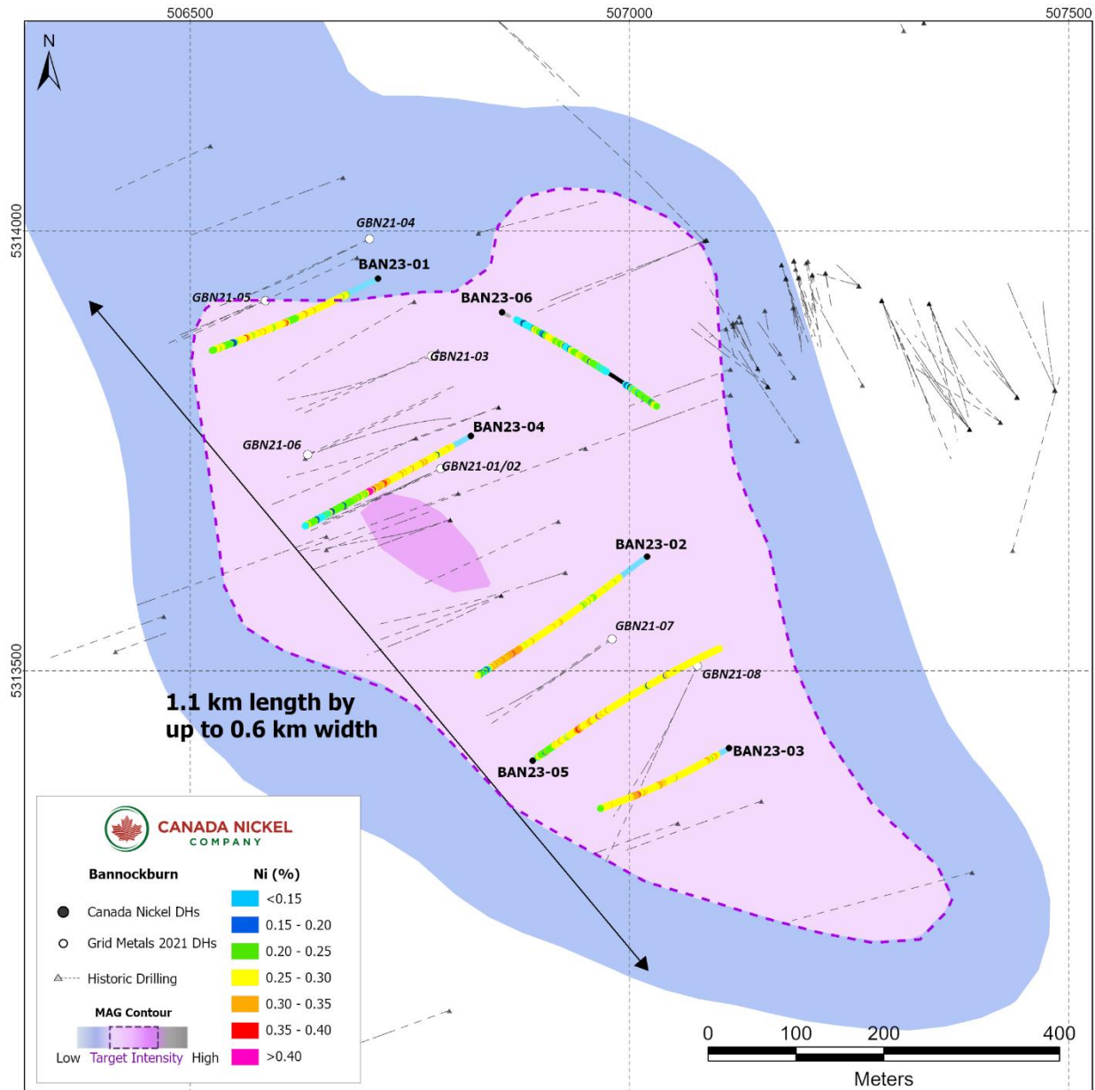
Abbildung 1 - Zone Bannockburn "B" - CNC-Bohrlöcher über der magnetischen Gesamtintensität.
