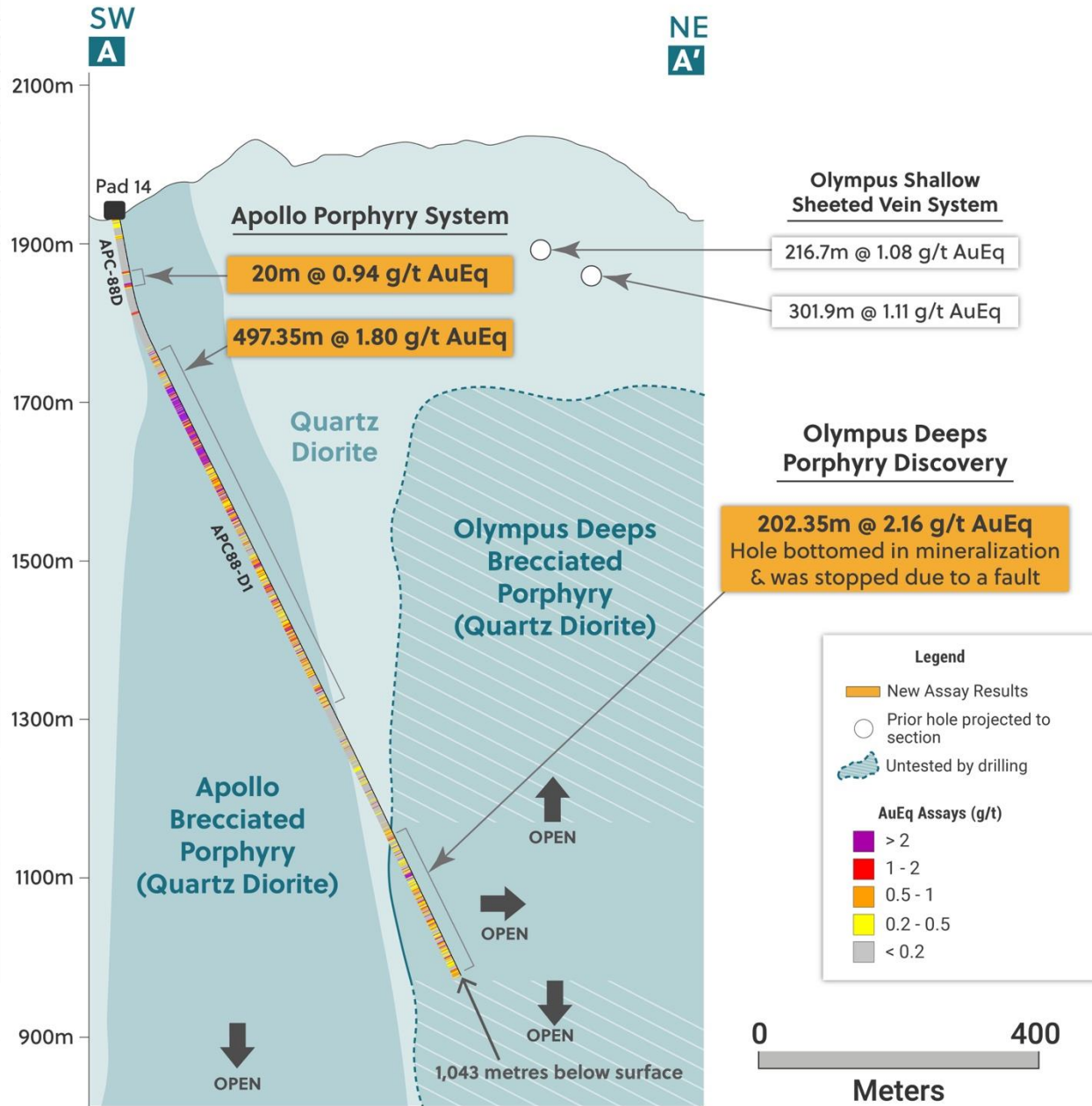
Abbildung 4: Querschnitt mit den Bohrungen APC-88D und APC88-D1
