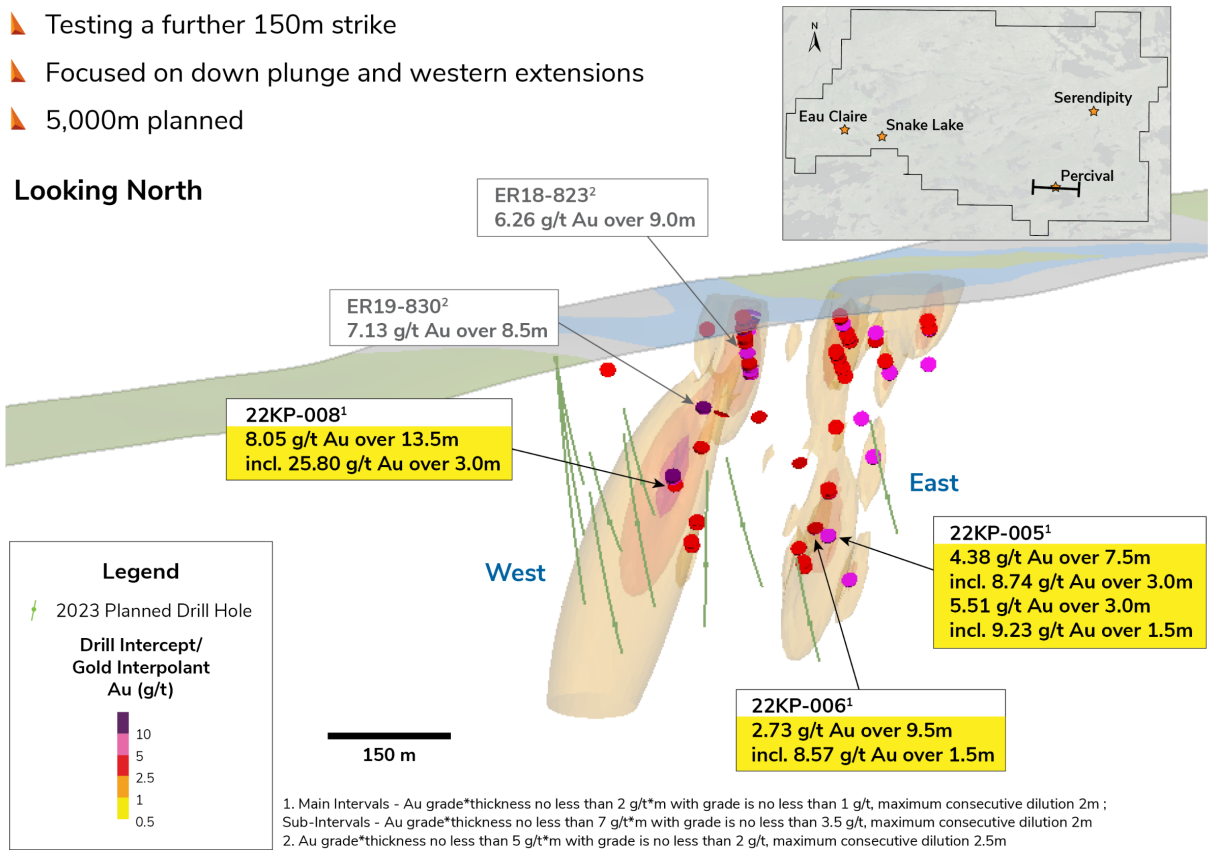
Abbildung 1: Langer Schnitt von Percival, der die Standorte der für 2023 vorgeschlagenen Bohrlöcher im Verhältnis zu den Abschnitten von 2022 und den historischen Bohrungen zeigt.
