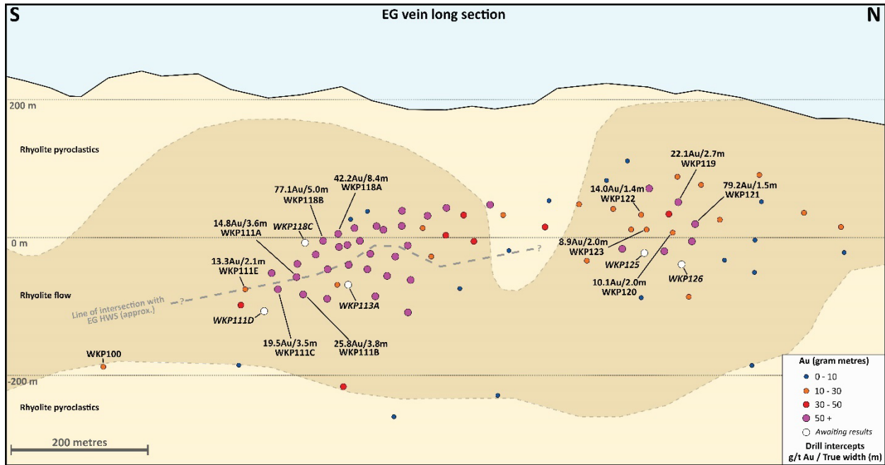
Abbildung 3: Längsschnitt der EG-Ader-Bohrschritte (neue Bohrlöcher beschriftet)
