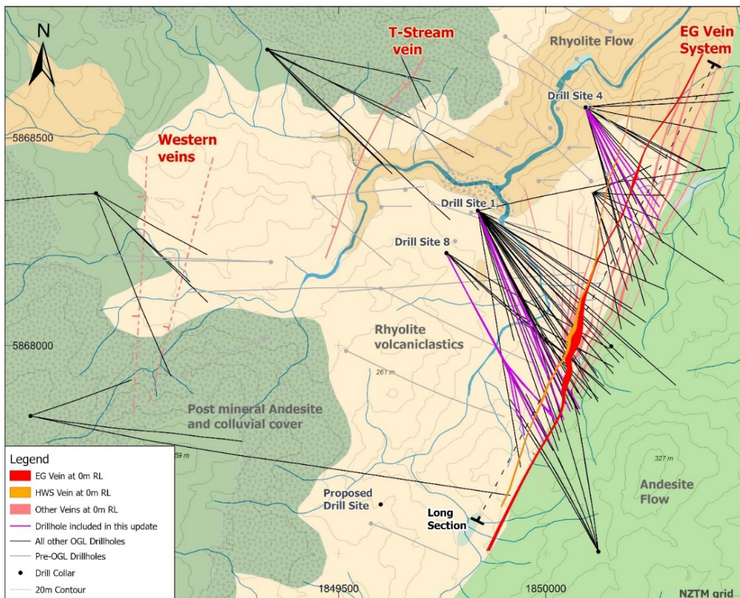
Abbildung 2: Wharekirauponga - Planansicht der Geologie, Bohrspuren und Verteilung der Aderzonen
