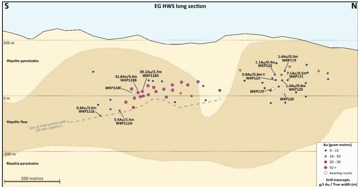
Abbildung 4: Längsschnitt durch die Ader EG HWS mit Hervorhebung der neuen Bohrungen
