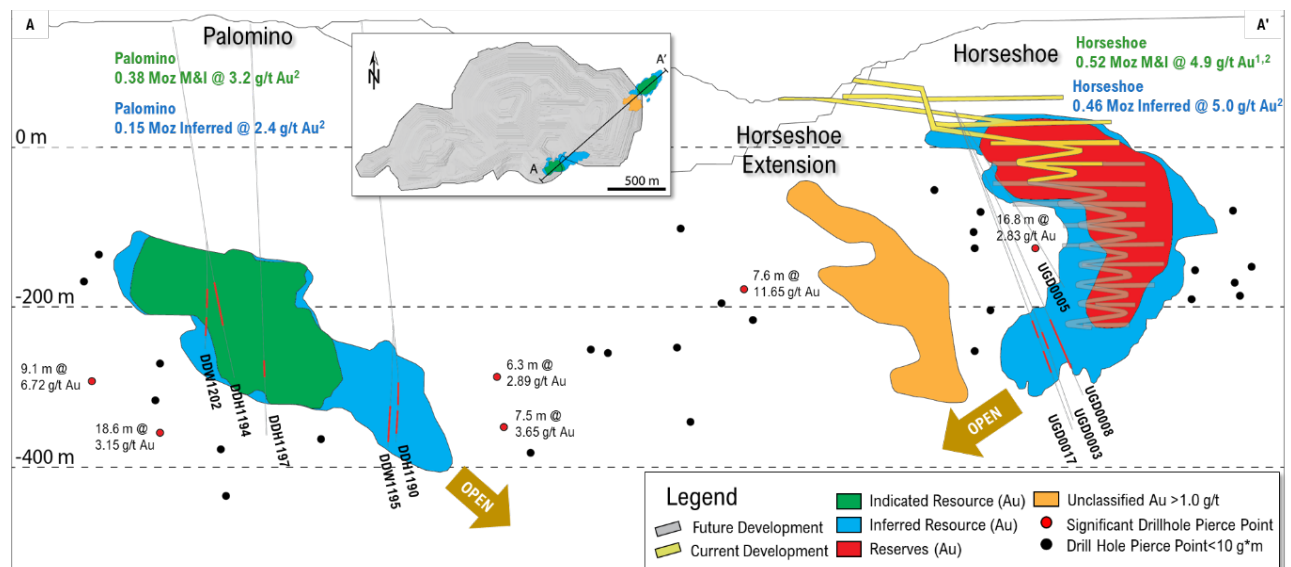
Abbildung 1: Längsschnitt (Blick nach Nordwesten) mit Palomino und Horseshoe und neuen Bohrlochergebnissen
