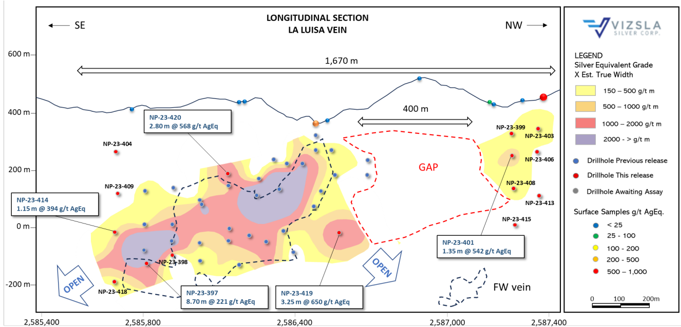
Abbildung 2: Längsschnitt durch die Ader La Luisa.
