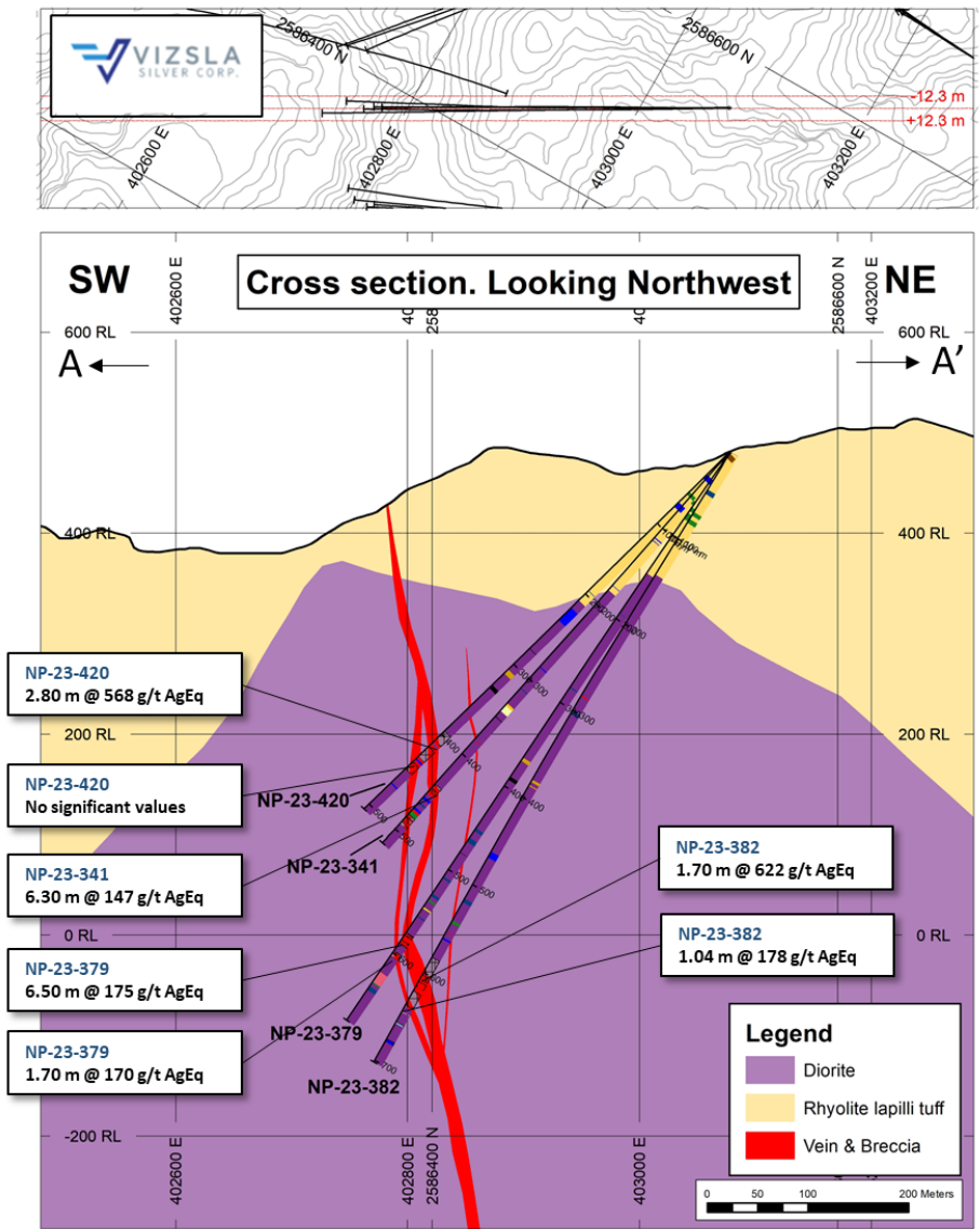
Abbildung 3: Längsschnitt durch die Footwall Ader bei La Luisa.
