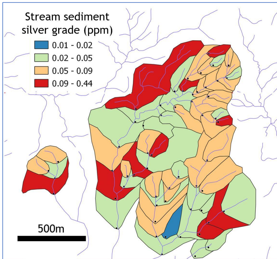
Abbildung 2. Karte mit dem Silbergehalt der Einzugsgebiete hinsichtlich jeder Entnahmestelle der Flusssedimente im epithermalen Zielgebiet Apai.
