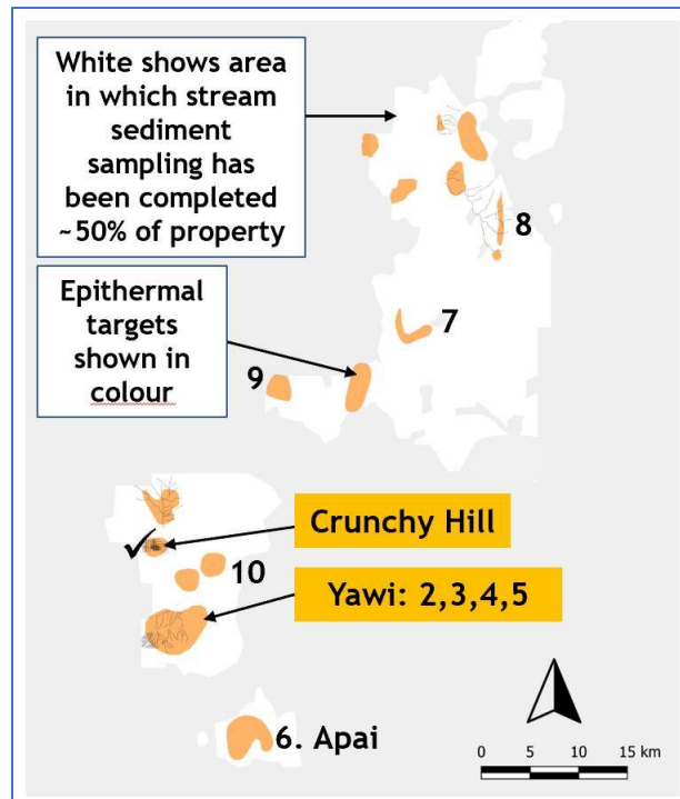
Abbildung 1. Die Karte zeigt die Ausdehnung der Flusssedimentprobenahme auf dem Projekt Lost Cities - Cutucu (weißer Bereich) mit Lage der epithermalen Ziele für Gold und Silber (in Farbe dargestellt). Die Zahlen neben den Zielbereichen beziehen sich auf die aktuelle Rangfolge der Erkundungsbohrungen.
