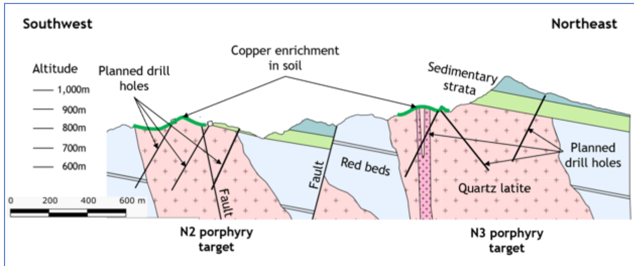
Abbildung 1. Querschnitt (vertikaler Schnitt) durch die Tsenken-Ziele N2 und N3 zur Veranschaulichung des Explorationskonzepts, das im Rahmen des Erkundungsbohrprogramms getestet werden soll.
