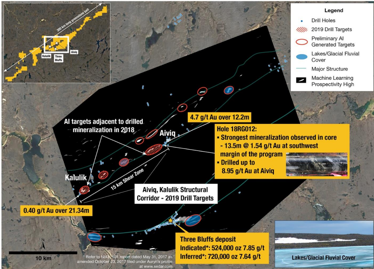
Abbildung 1: Veranschaulicht die Ziele, die mithilfe des maschinellen Lernens entlang des tektonischen Korridors Kalulik – Aiviq generiert wurden. Dies wird die Basis des Sommerbohrprogramms 2019 bilden.
