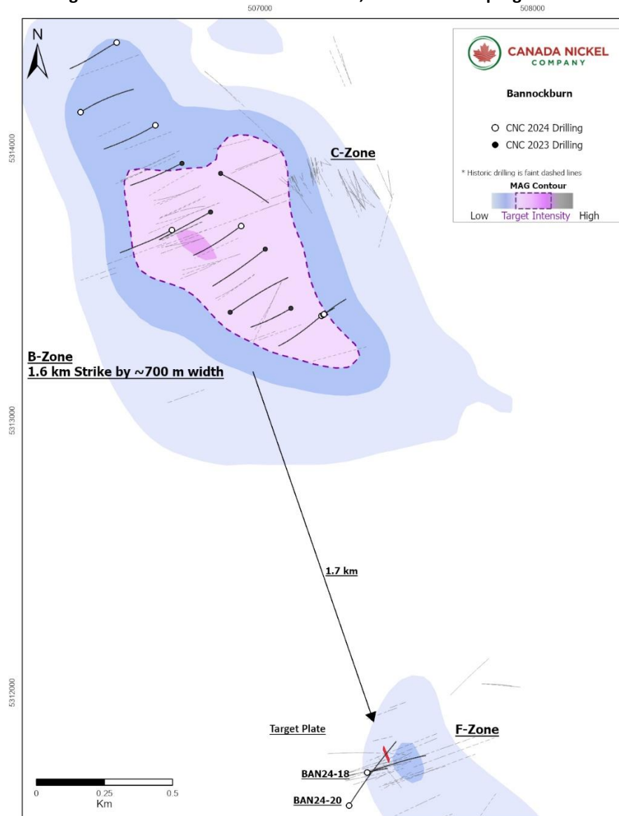
Abbildung 1 - Bannockburn B-Zone und F-Zone, laufendes Bohrprogramm.
