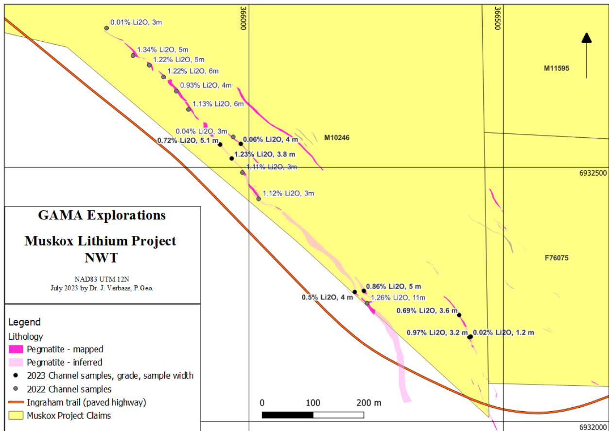
Abbildung 1. Der CM-1-Pegmatit innerhalb des Muskox-Lithiumprojekts in den Northwest Territories, der den Standort der Schlitzproben und Untersuchungsergebnisse zeigt.
