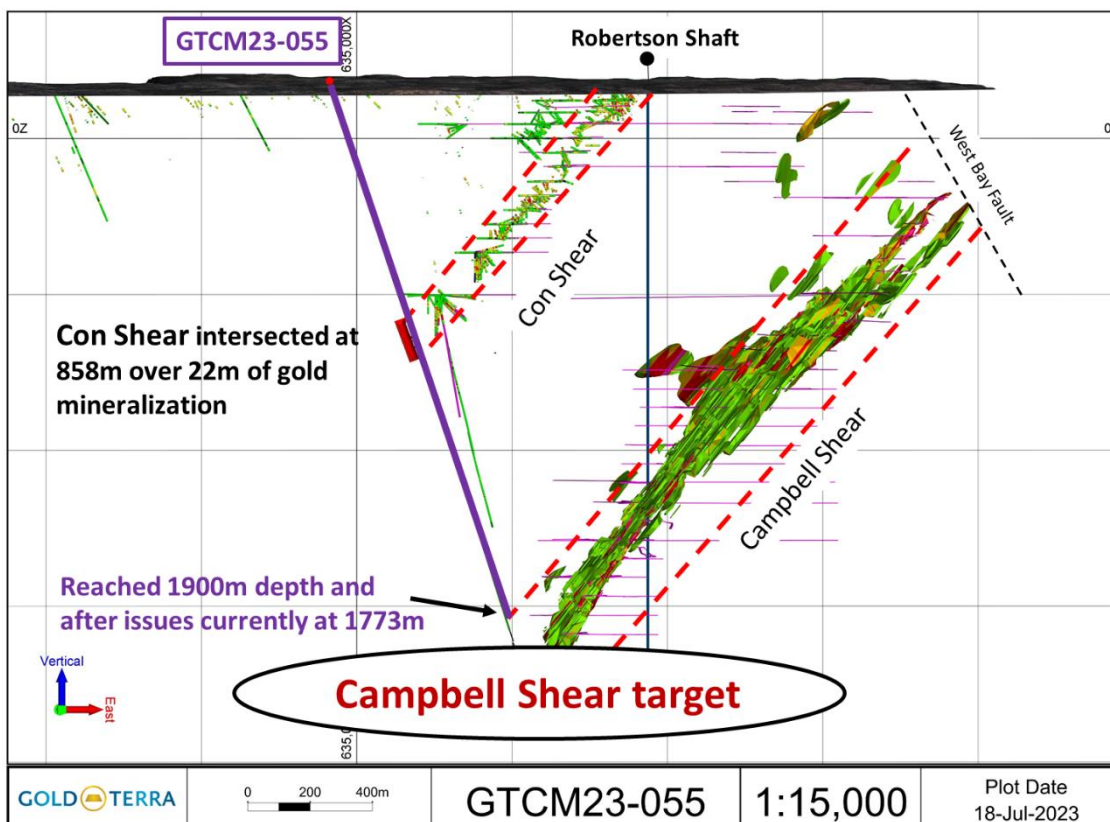
Abbildung 1 - Querschnitt mit Blick nach Norden, der das Bohrloch GTCM23-055 zeigt, das die Scherflächen Con und Campbell unterhalb des ehemaligen Untertagebaus der Mine Con ansteilt.
