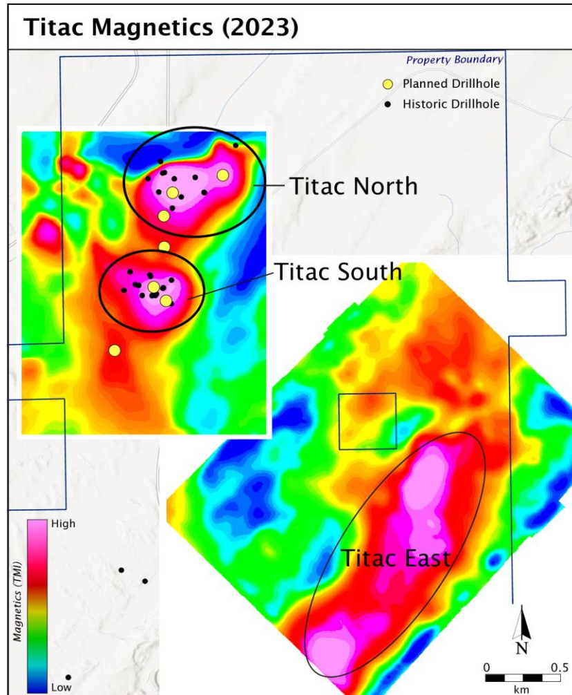
Abbildung 2. Magnetismus (Drohne) in Titac South, Titac North und Titac East. Eine neue VTEM-Untersuchung wird die Auflösung und das/die Bohrziel/e in Titac East verfeinern.
