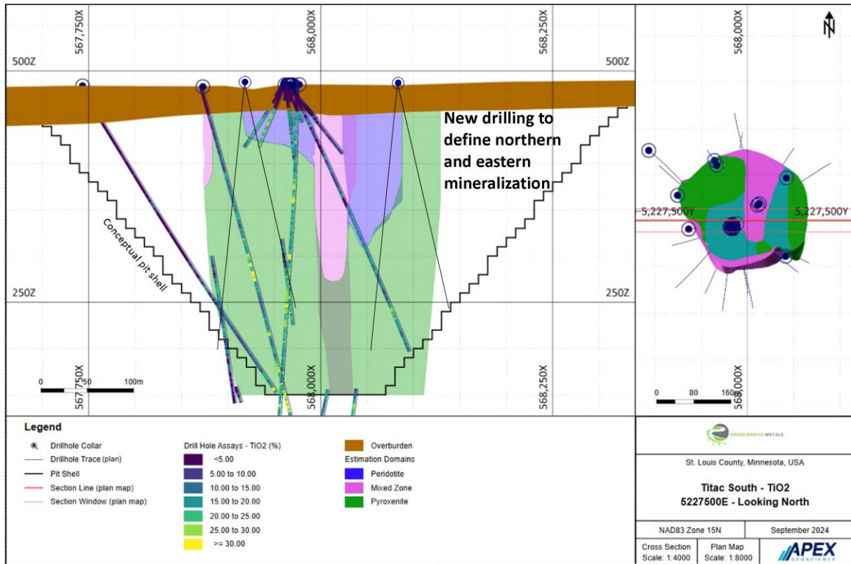
Abbildung 1. Querschnitt der Lagerstätte Titac South bei 5227500 m E mit Kennzeichnung von \text{TiO}_2 (%) mit Blickrichtung Norden. Darstellung der potenziellen Standorte für neue Kernbohrungen (schwarze Linien).
