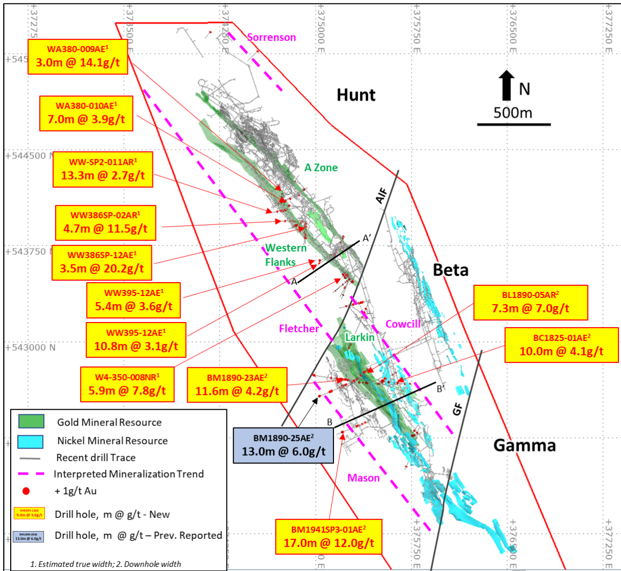
Abbildung 1: Planansicht von Beta Hunt mit den jüngsten Goldergebnissen für den Zeitraum 24. Juli bis 13. Oktober 2022
