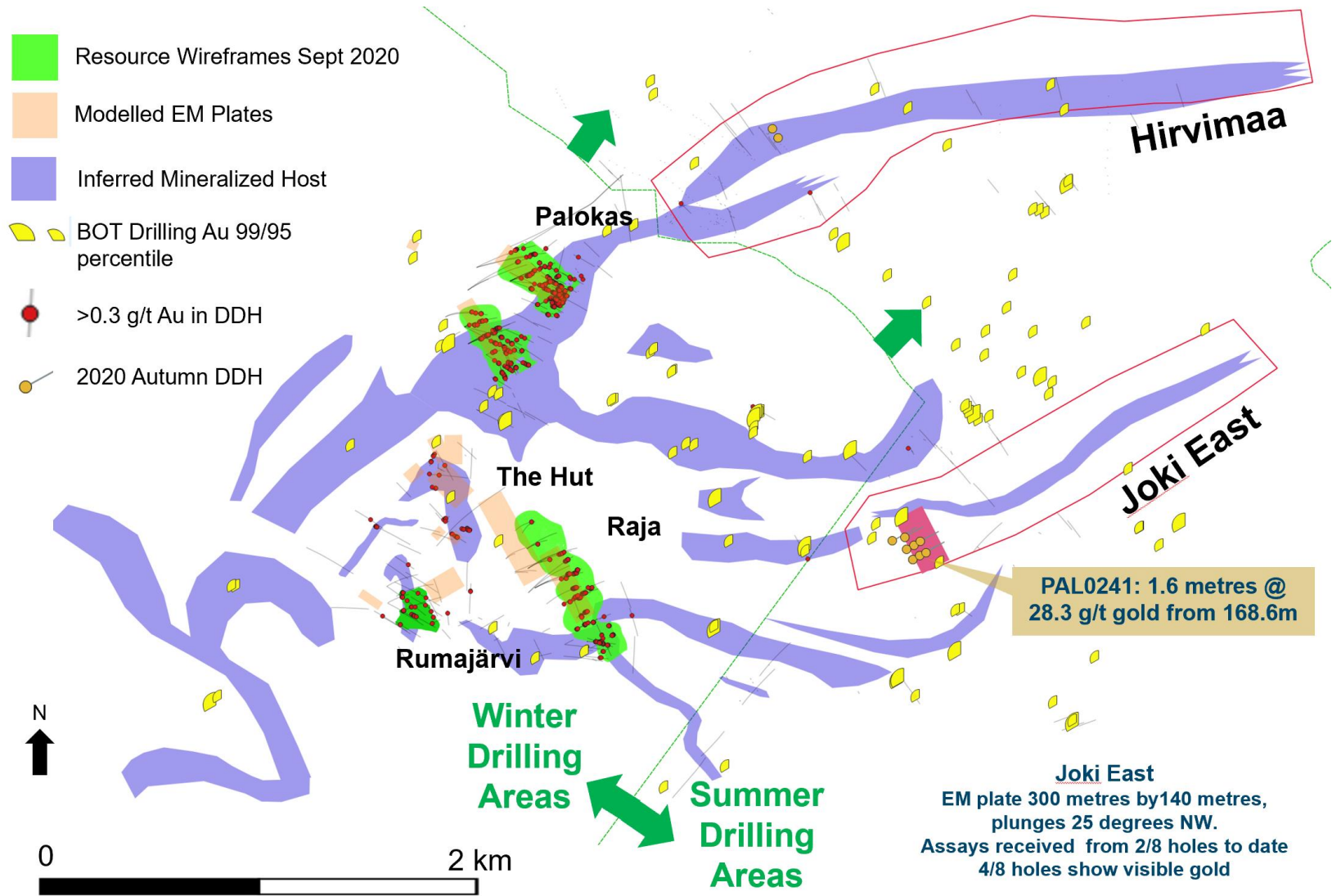
Abbildung 1: Lageplan des Projekts Rajapalot mit im Rahmen des Herbstbohrprogramms 2020 niedergebrachten Bohrungen, leitenden TEM-Platten in Joki East, Drahtgittermodellen der Ressourcen aus der Ressourcenschätzung vom September 2020, modellierten EM-Platten der Base-of-Till Bohrungen (BOT, Bohrungen ab der Basis des Geschiebemergels) mit anomalen Gehalten und den im Sommer genehmigten Zielgebieten East Joki und Hirvima.aa.
