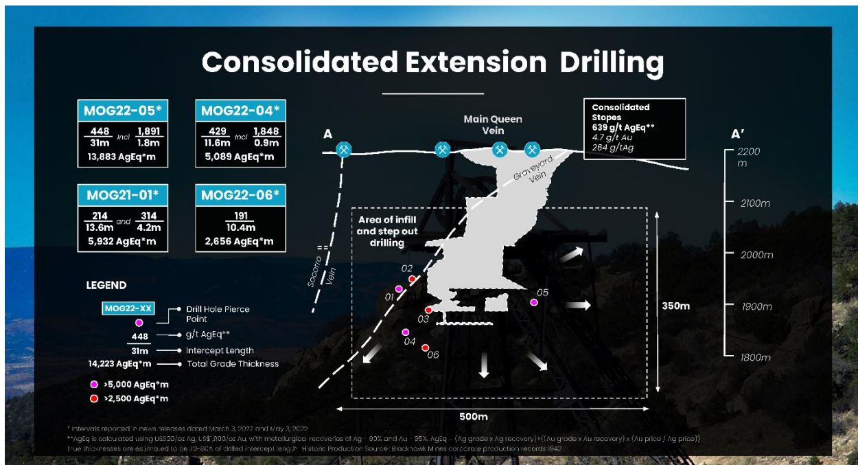
Abbildung 3: Konsolidierte Erweiterung Langschnitt
