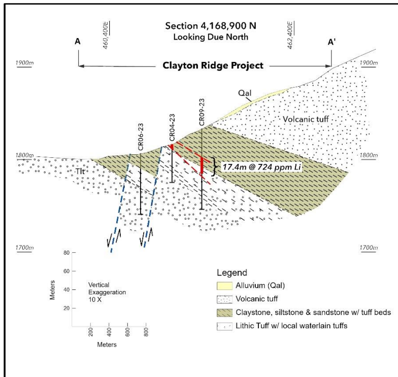
Abbildung 2. Geologischer Abschnitt A-A', der den nach Osten einfallenden, Li-haltigen Tonstein zeigt, der in den Löchern CR04, -06 und -09-23 beobachtet wurde. Die Lage des Abschnitts ist in Abbildung 1 dargestellt. Topografie und Mächtigkeit wurden durch 10-fache vertikale Überhöhung verstärkt.
