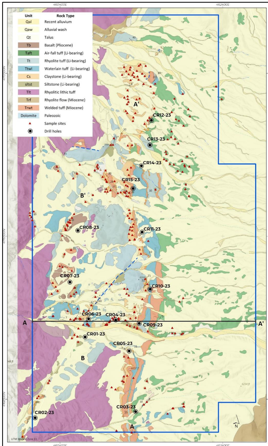
Abbildung 1. Geologische Karte des Clayton Ridge Basin innerhalb des USCM-Geländes (blaue Linie) mit den Standorten der Kernbohrungen 2023. Der Abschnitt A-A' ist in Abbildung 2 dargestellt.
